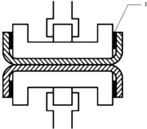
图 4 定量分析法(方法 B)中试样在铝制夹具中的固定方法
