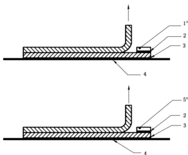
图 1 定性分析法(方法 A)试样组合方法
